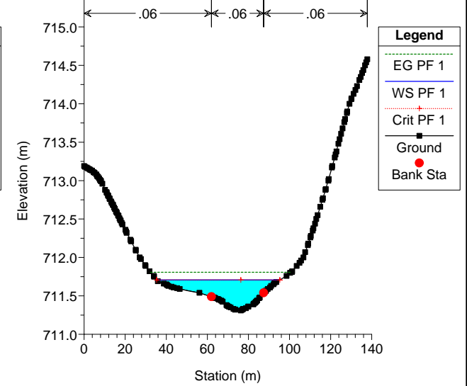
ARROYO LARIJA Plan: SITUACION ACTUAL 02 Geom: SITUACION ACTUAL 02 Flow: CAUDAL 500 River = ARROYO Reach = LARIJA RS = 271
