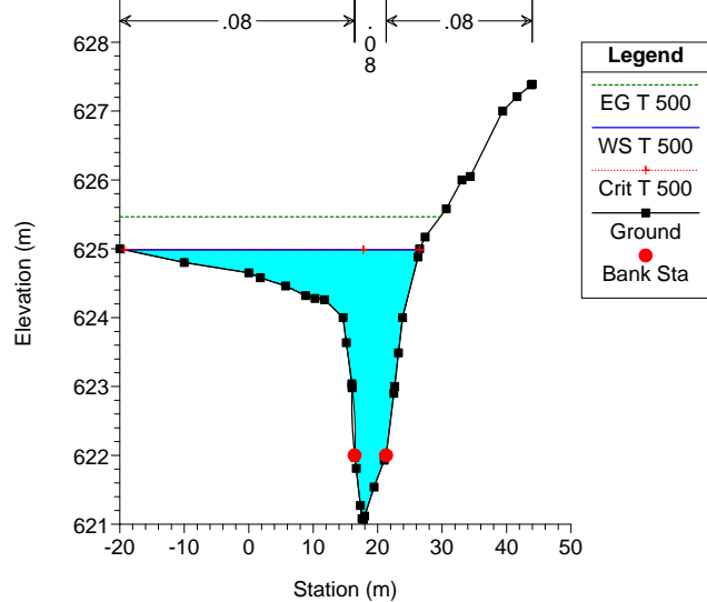
FUENTE DE LA VILLA Plan: SITUACION ACTUAL 01 Geom: SITUACION ACTUAL Flow: CAUDAL 500 River = FUENTE Reach = VILLA RS = 97.5*
