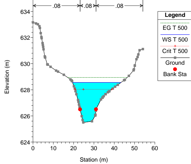
FUENTE DE LA VILLA Plan: SITUACION ACTUAL 01 Geom: SITUACION ACTUAL Flow: CAUDAL 500 River = FUENTE Reach = VILLA RS = 251
