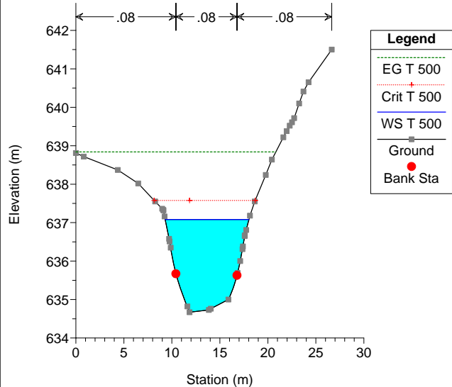
FUENTE DE LA VILLA Plan: SITUACION ACTUAL 01 Geom: SITUACION ACTUAL Flow: CAUDAL 500 River = FUENTE Reach = VILLA RS = 544.333*
