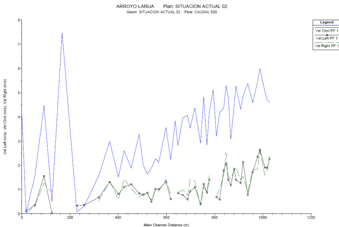
Ilustración 13. Velocidades
