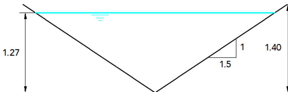
Ilustración 19. Propuesta acondicionamiento en tramo cuneta
