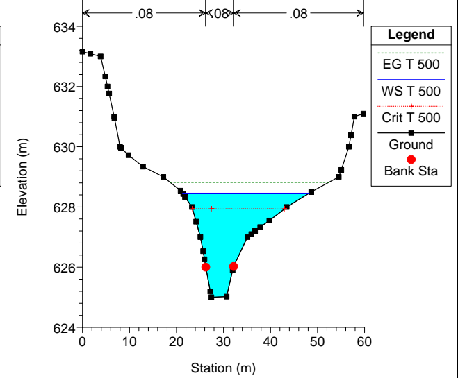
FUENTE DE LA VILLA Plan: SITUACION ACTUAL 01 Geom: SITUACION ACTUAL Flow: CAUDAL 500 River = FUENTE Reach = VILLA RS = 243.666*
