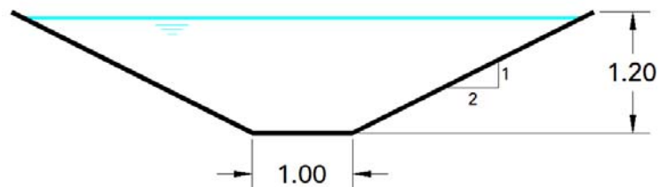
Ilustración 12. Croquis Propuesta 1
