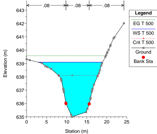
FUENTE DE LA VILLA Plan: SITUACION ACTUAL 01 Geom: SITUACION ACTUAL Flow: CAUDAL 500 River = FUENTE Reach = VILLA RS = 537.666*
