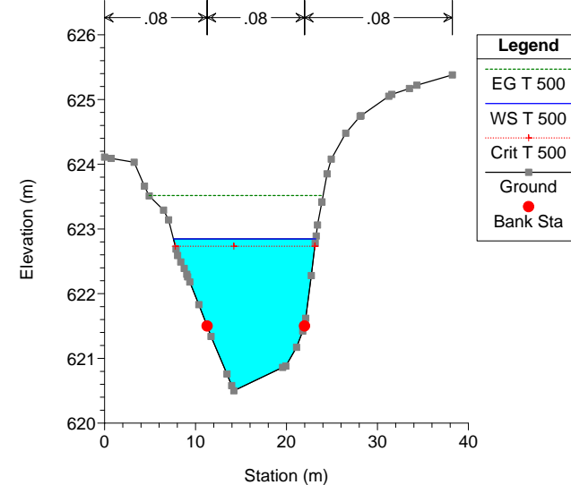
FUENTE DE LA VILLA Plan: SITUACION ACTUAL 01 Geom: SITUACION ACTUAL Flow: CAUDAL 500 River = FUENTE Reach = VILLA RS = 90.*
