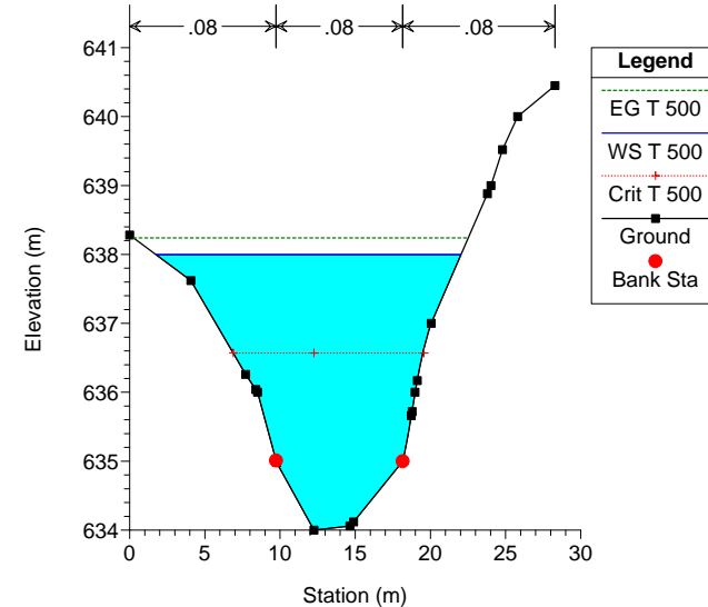
FUENTE DE LA VILLA Plan: SITUACION ACTUAL 01 Geom: SITUACION ACTUAL Flow: CAUDAL 500 River = FUENTE Reach = VILLA RS = 531
