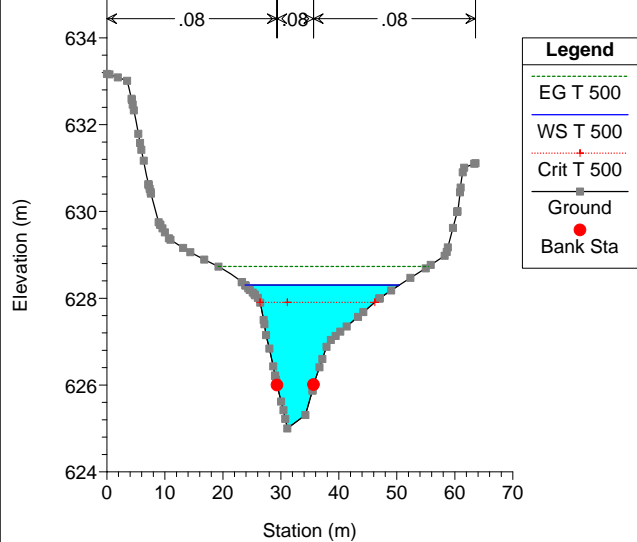
FUENTE DE LA VILLA Plan: SITUACION ACTUAL 01 Geom: SITUACION ACTUAL Flow: CAUDAL 500 River = FUENTE Reach = VILLA RS = 256.5*
