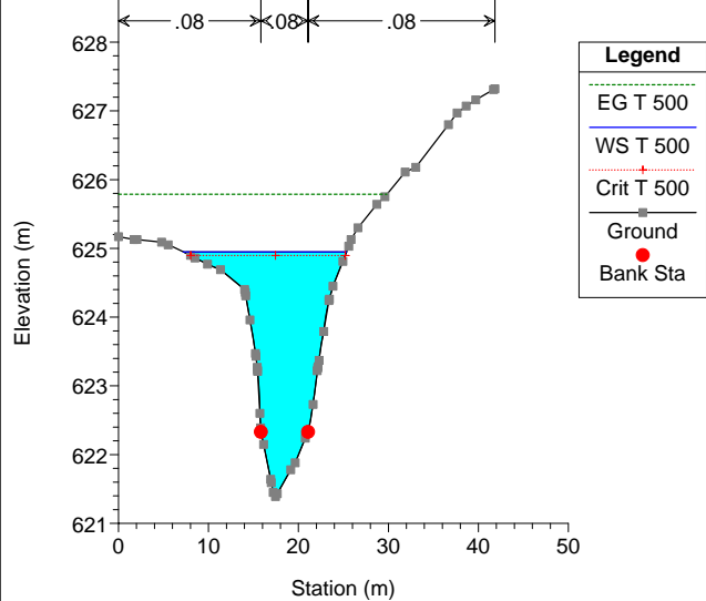
FUENTE DE LA VILLA Plan: SITUACION ACTUAL 01 Geom: SITUACION ACTUAL Flow: CAUDAL 500 River = FUENTE Reach = VILLA RS = 105
