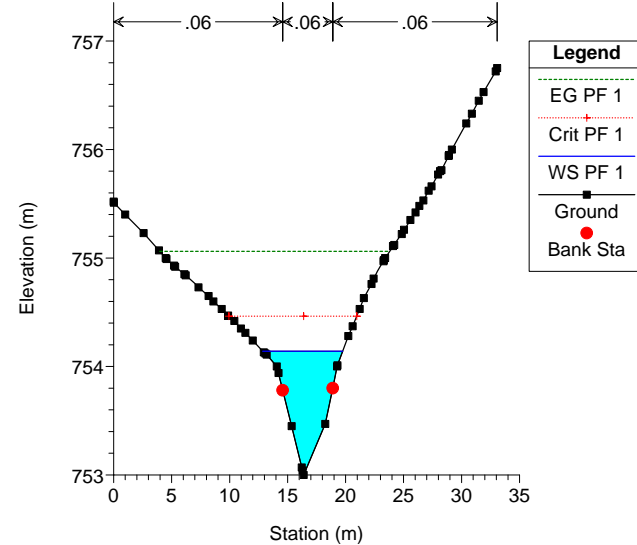
ARROYO LARIJA Plan: SITUACION ACTUAL 02 Geom: SITUACION ACTUAL 02 Flow: CAUDAL 500 River = ARROYO Reach = LARIJA RS = 879
